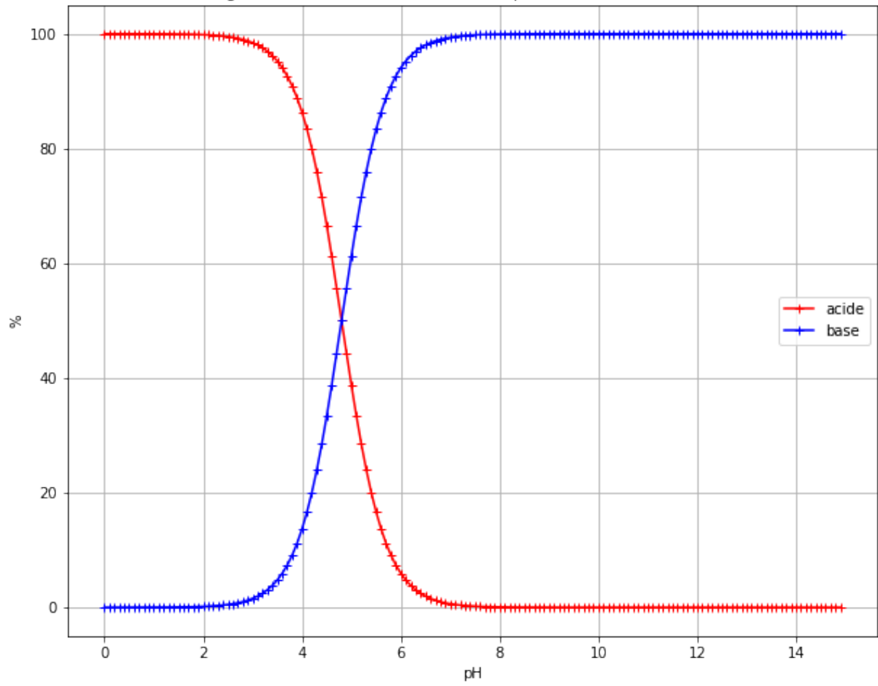
Diagramme de distribution d'un couple acide faible/base faible
